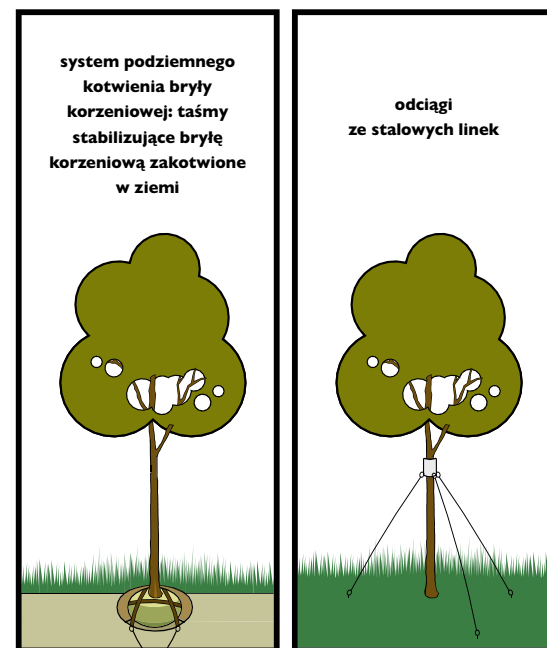
INNE SPOSOBY STABILIZACJI DRZEWA
