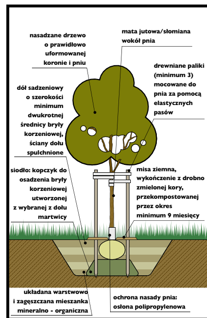
SCHEMAT SADZENIA ORAZ STABILIZACJI DRZEWA
