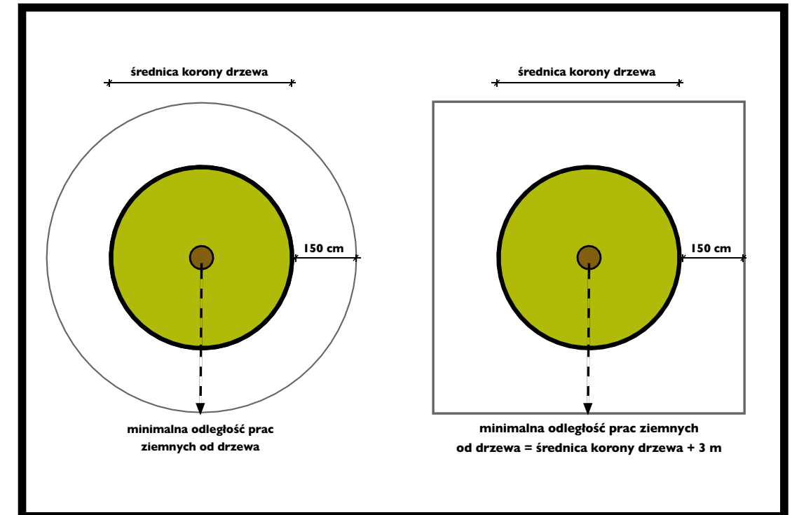
SPOSÓB WYZNACZANIA GRANIC STREFY OCHRONNEJ DLA POJEDYNCZEGO DRZEWA ORAZ DLA GRUPY ROŚLIN
