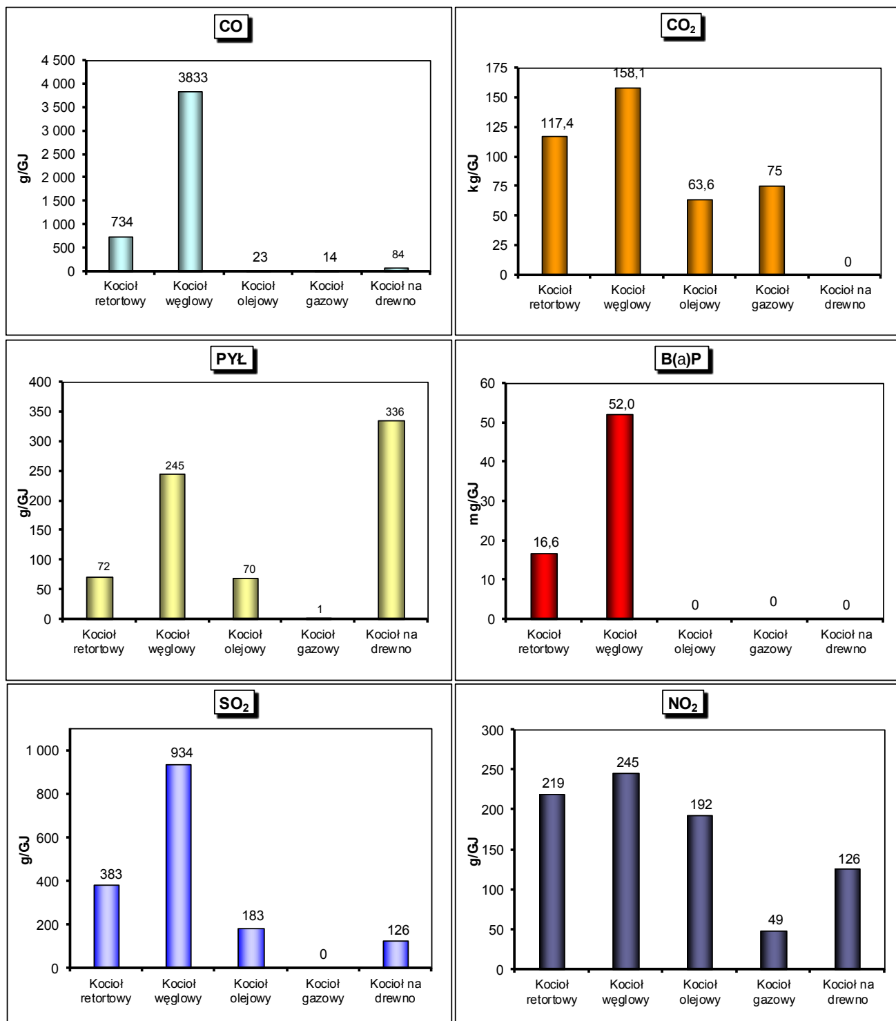
Rysunek 3.3. Porównanie emisji zanieczyszczeń powstających przy spalaniu paliw do celów grzewczych przy produkcji 1 GJ ciepła użytkowego (z uwzględnieniem sprawności energetycznej urządzeń grzewczych)
